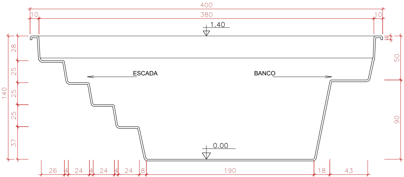
CORTE LONGITUDINAL SEM ESCALA
