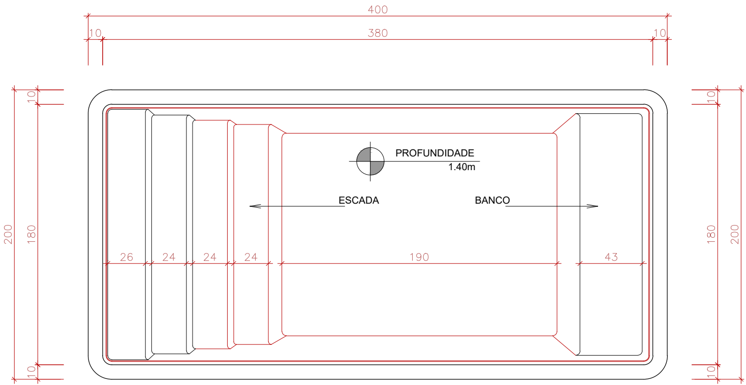
PLANTA BAIXA SEM ESCALA
