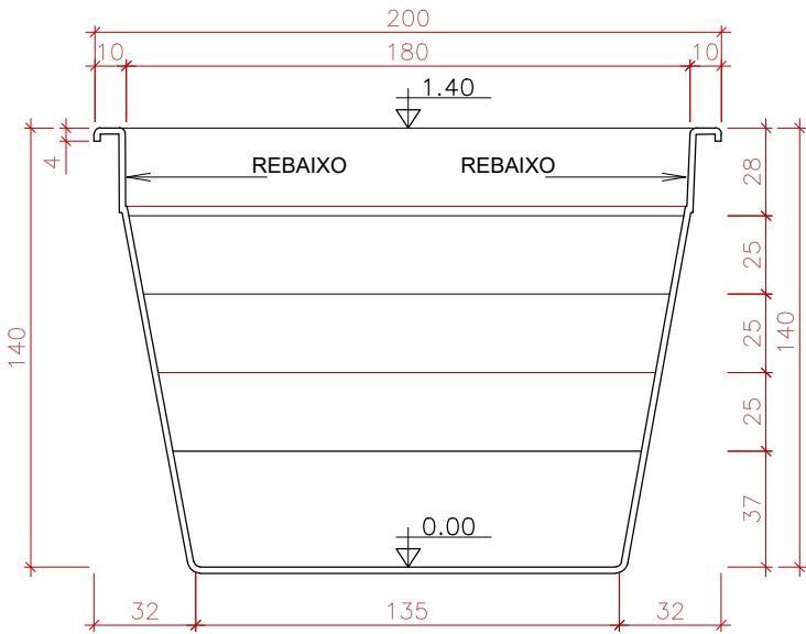
CORTE TRANSVERSAL SEM ESCALA
